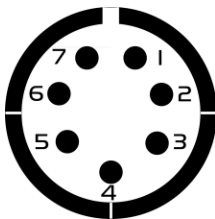
Binder Stecker 711-7 Lötansicht
