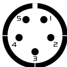
711-5 Lötansicht
