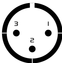
711-3 Lötansicht
