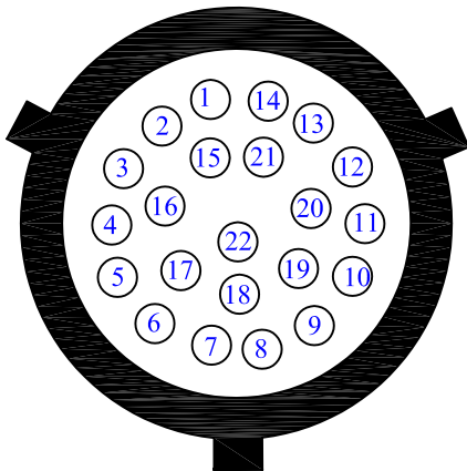
Vista del connettore Deutsch dallato inserzione contatti.
