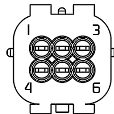
EURO5, männlich, Steckansicht
