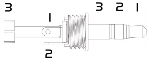
Klinke 2,5 mm, männlich, Lötansicht
